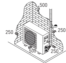
схема установки
