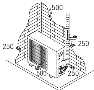
схема установки
