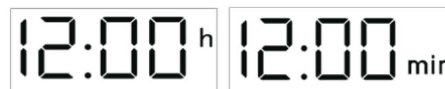
Настройка часов
