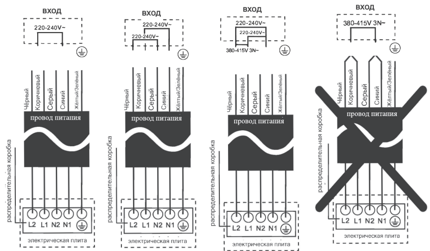
Метод соединения
