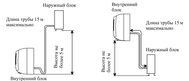
Схема установки
