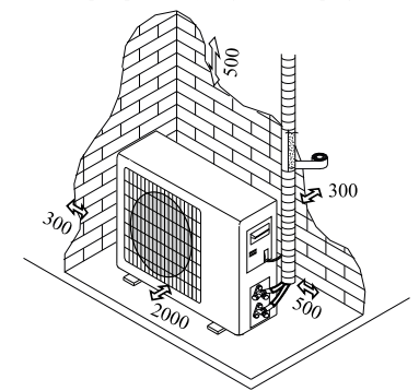
минимальное свободное пространство (мм) указано на рисунке
